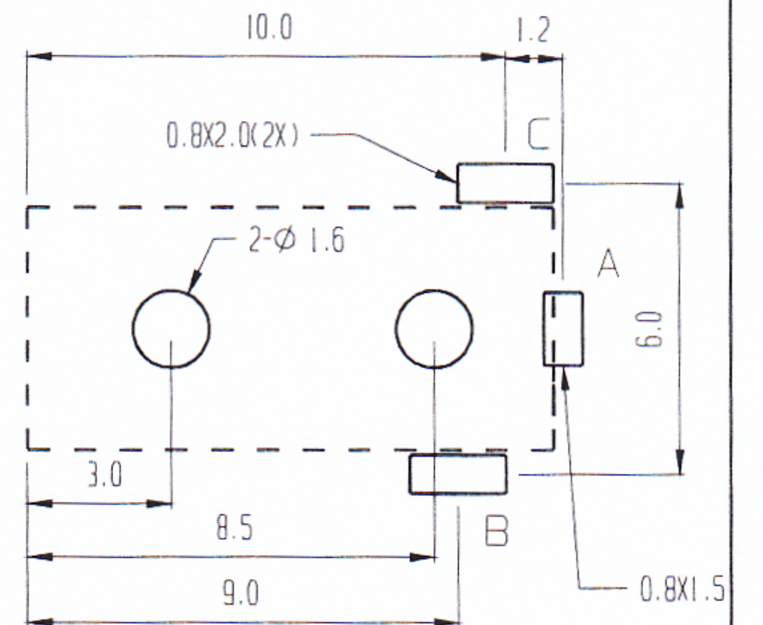
P.C.B. LAYOUT
